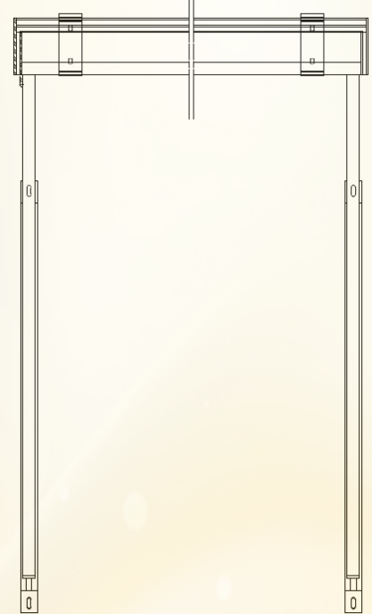
bevestiging kast door ophangprofiel fixation de caisson par profil de suspension
